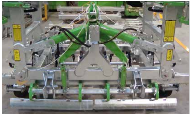
Voorraanzicht met schrapers
